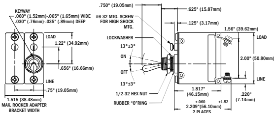
7312 COTS Metal Toggle
